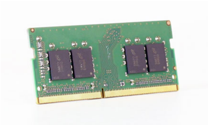
DIMM SO-DDR-4 16GB (DDR IV)
